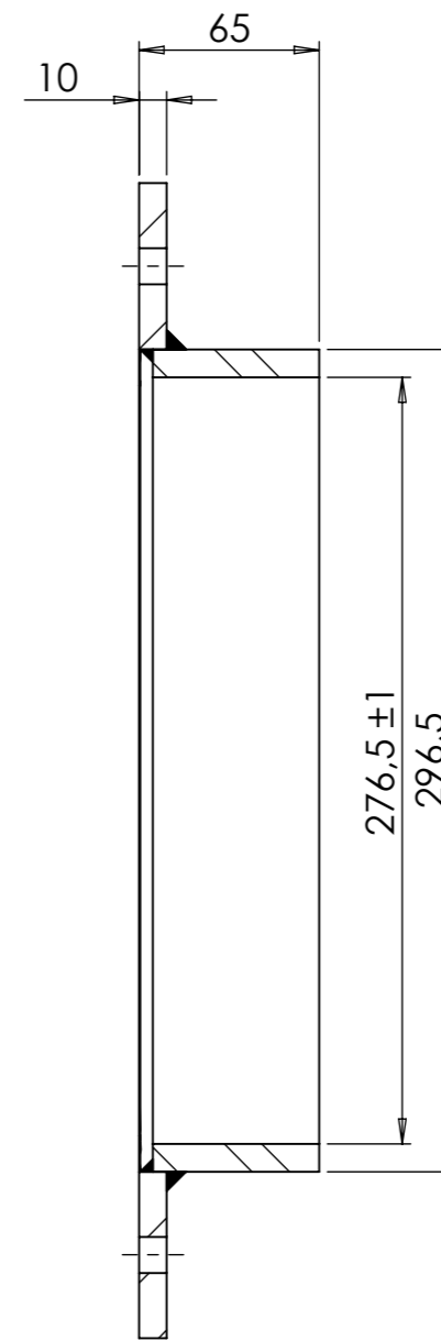
SECTION A-A
