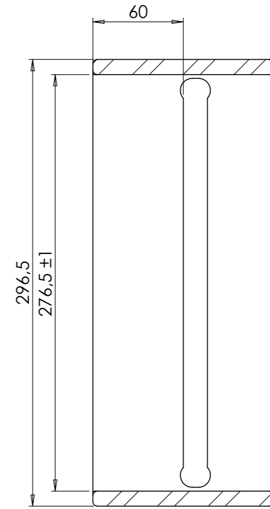
SECTION A-A
