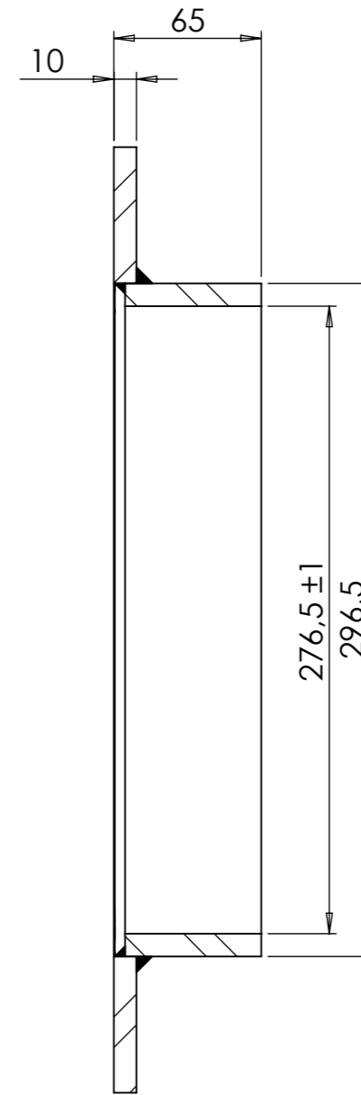
SECTION A-A
