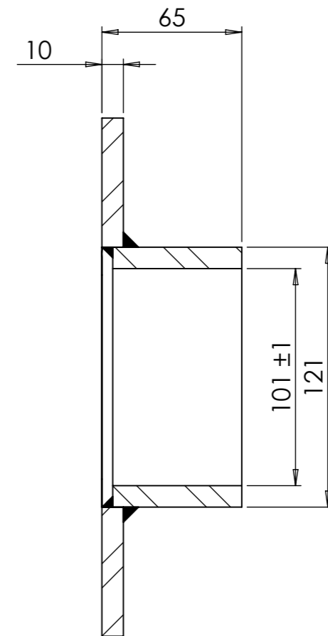
SECTION A-A
